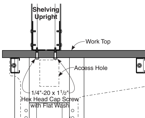
C-Leg Table
